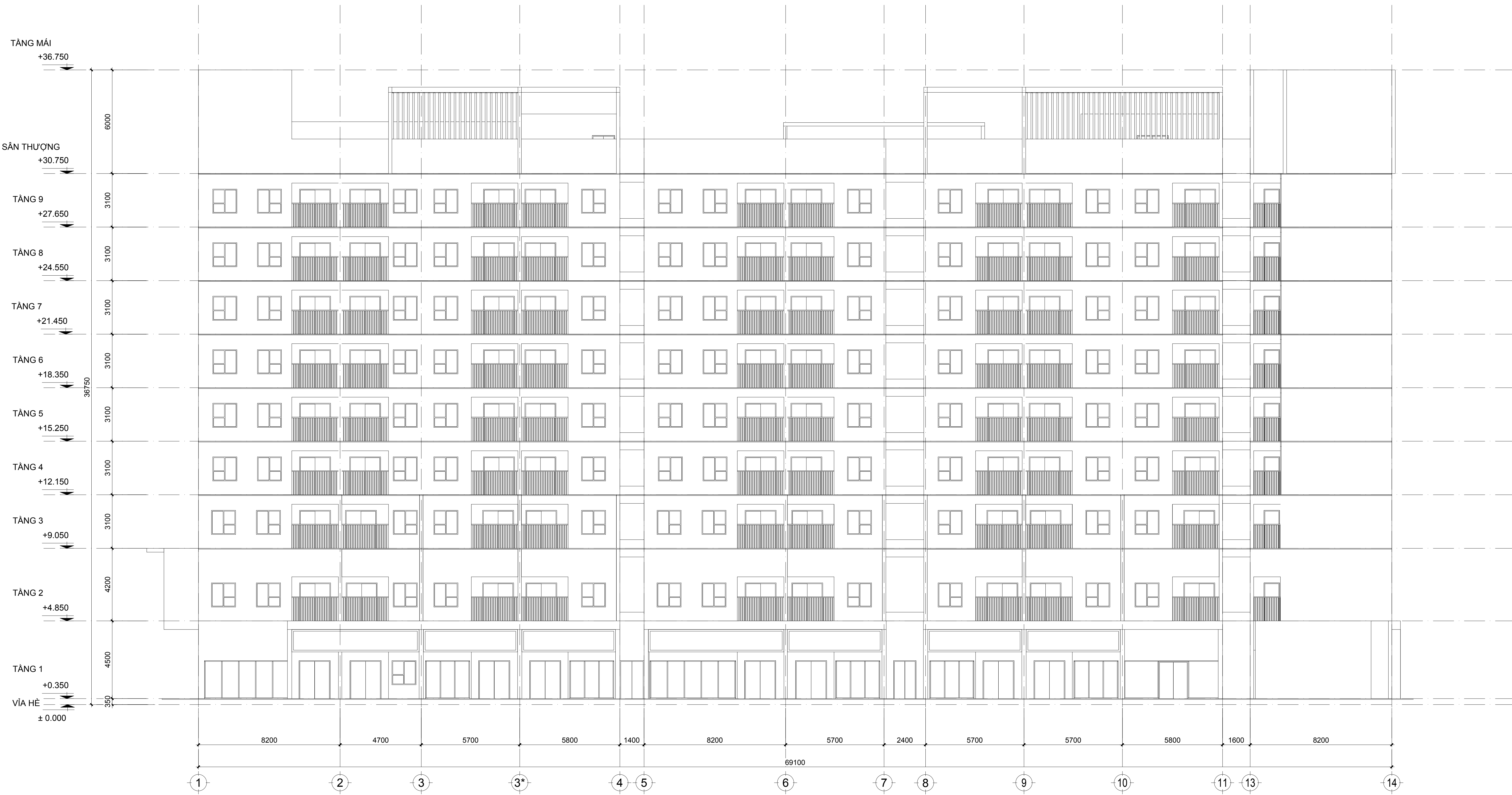
MẶT ĐỨNG TRỤC 1 - 14 TL:1/150 (KHỐI A)
